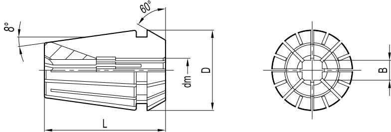
ER攻丝筒夹 ER Tapping Collet
