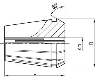
ER弹性筒夹 ER Collet
